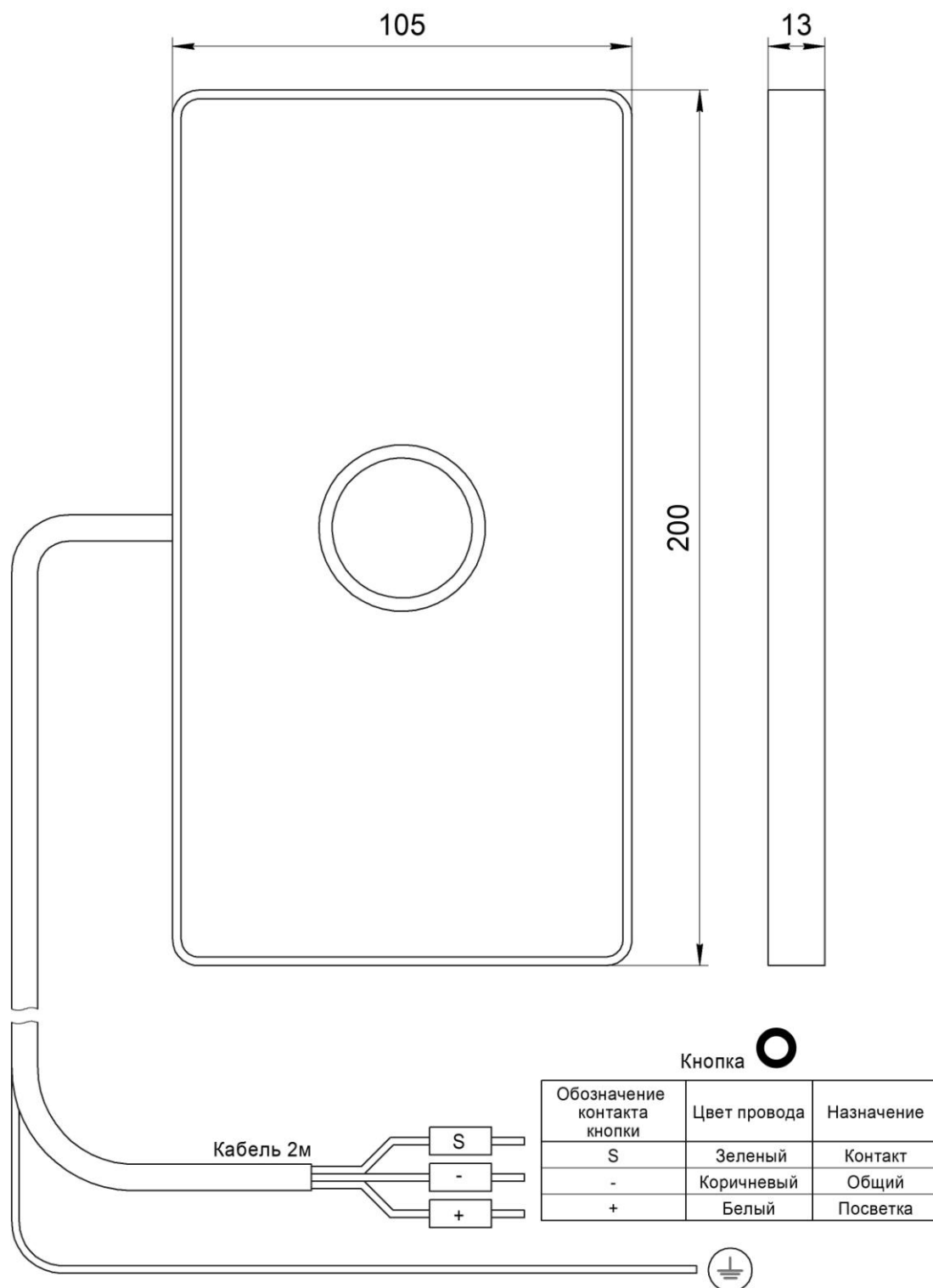
Рис.1 Внешний вид и габаритные размеры Вызывного поста МАЛАХИТ НШЕК.468381.060-01
